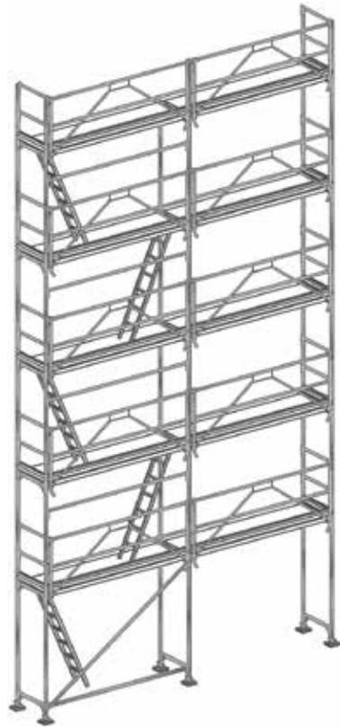
R200 FRAMESTEIGER 2 VELDEN
