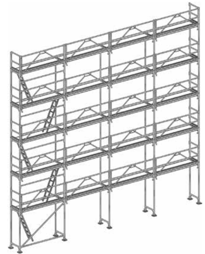
R200 FRAMESTEIGER 4 VELDEN
